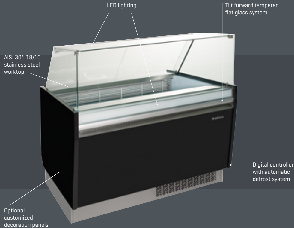
IDC-VBZ12
